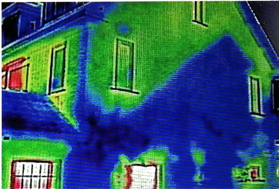
De warmtelekken in beeld van een woning in Bennebroek.
